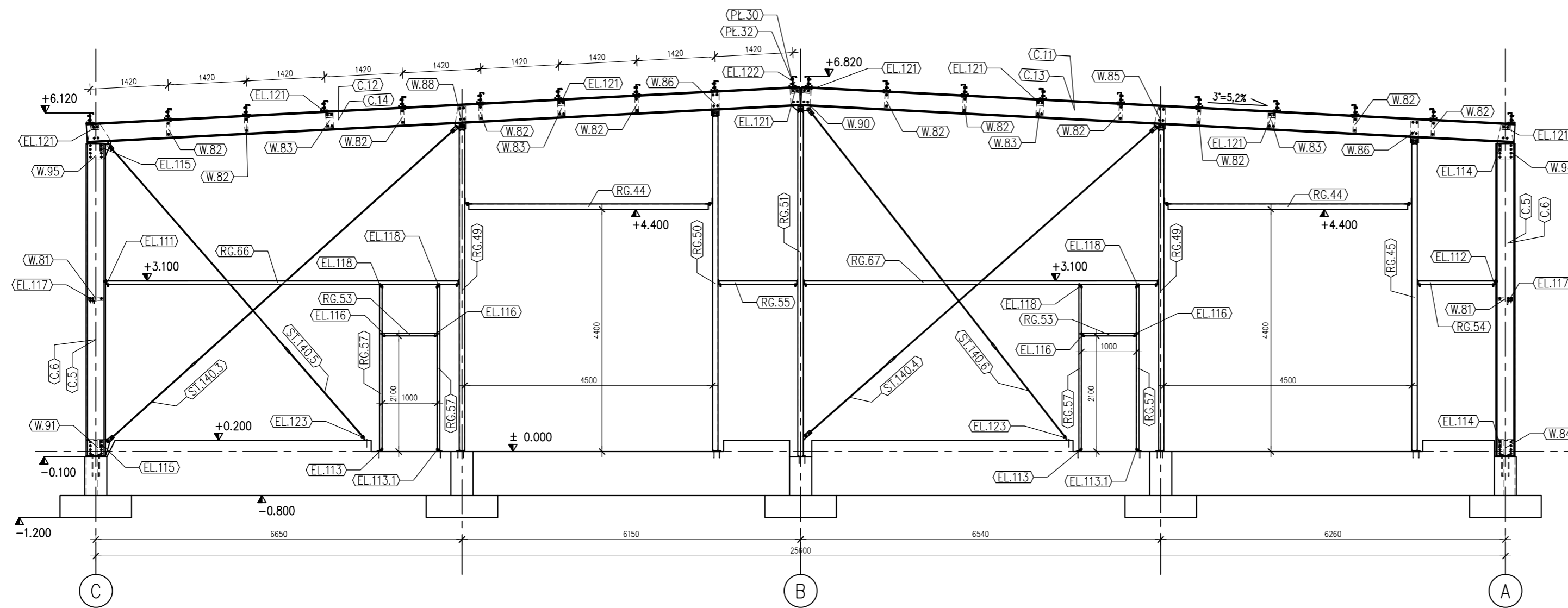
PRZEKRÓJ W OSI '1' (Sc1:50)
