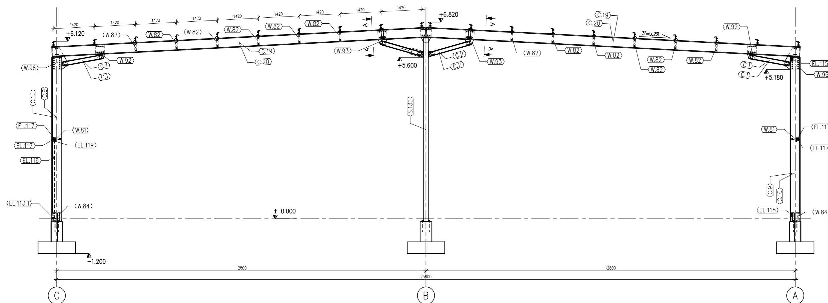
PRZEKRÓJ W OSI '4' (Sc1:50)
